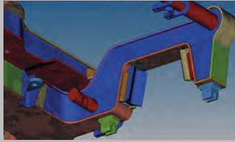
Bogie Frame Sonlu Elemanlar(FEA) Analiz Çalışmaları
