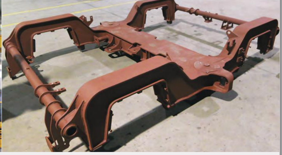
Bogie Frame Dayanım Testlerinde Kullanılacak Motorlu Bogie Üretimi
